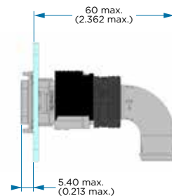
90° Indexable Chimney
